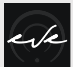
Web Pages
