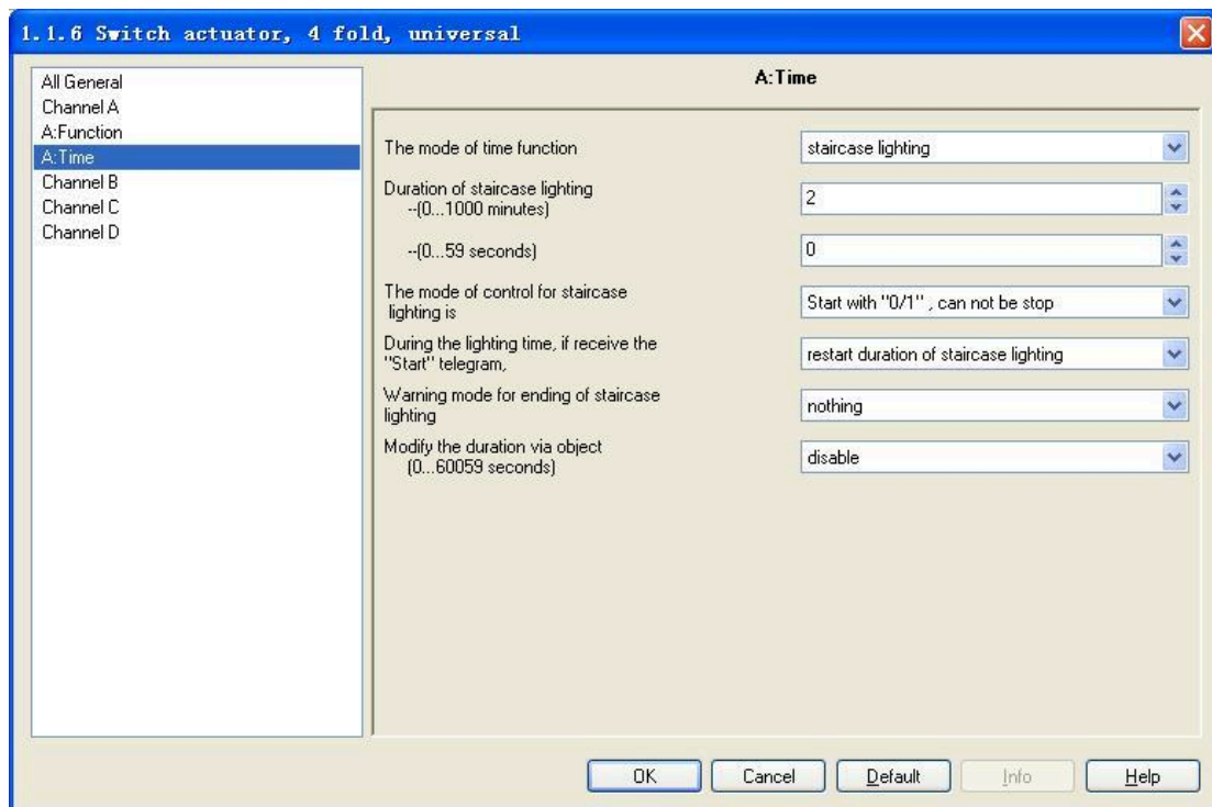
Fig. 7- Parameter window “X: Time-Staircase lighting”
