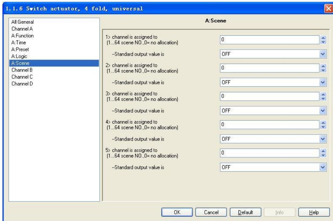
Fig.11 - Pparameter window “X: Scene”
