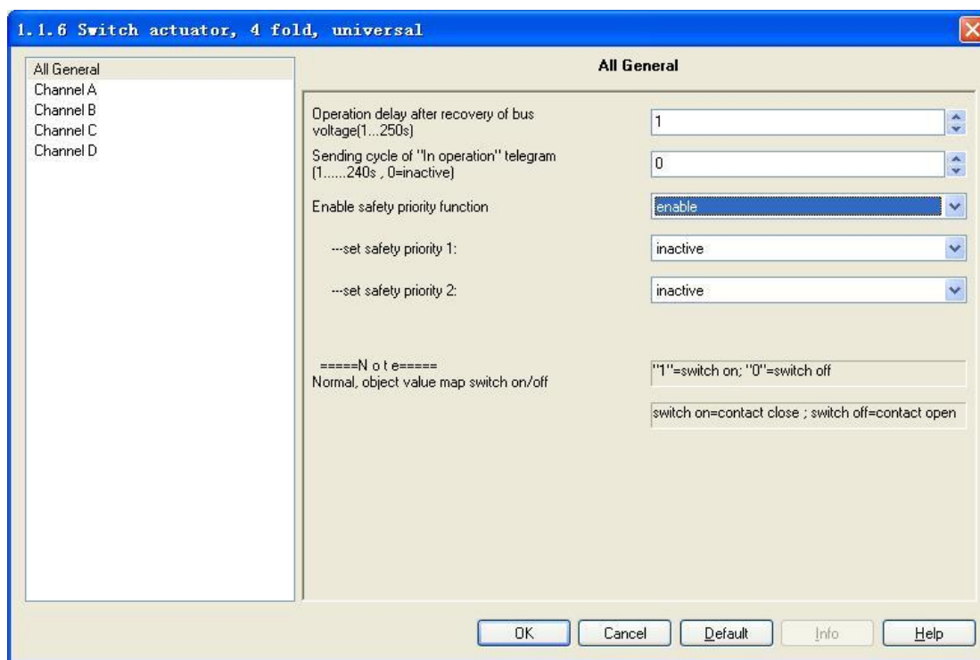
Fig.2 - Parameter window "Safety Priority"
