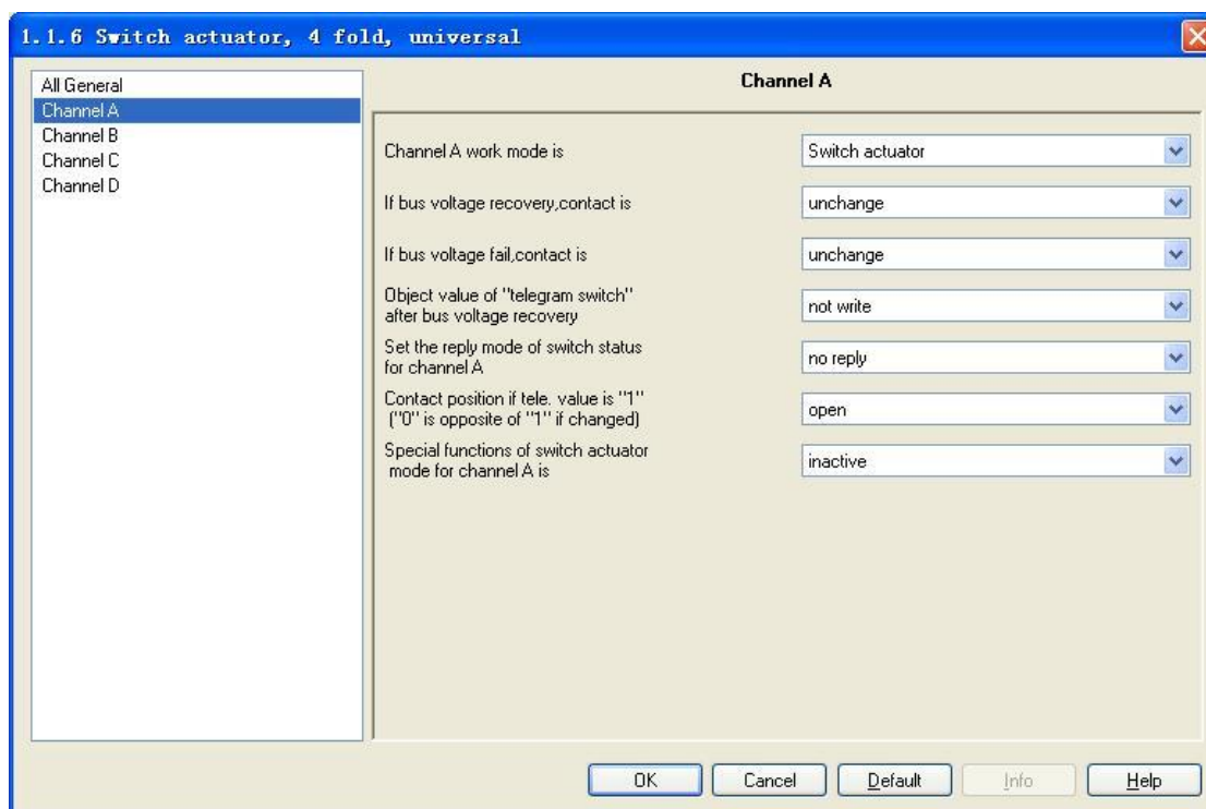
Fig.3 - Parameter window “Channel X”
