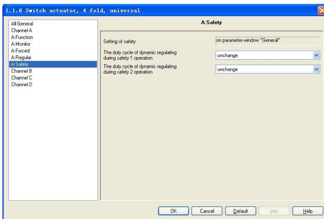
Fig.20 - Parameter window “X: Safety”
