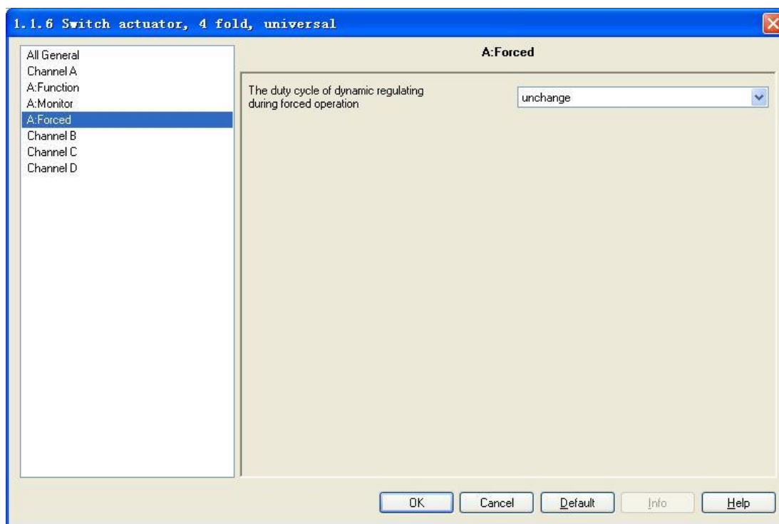
Fig.18 - Parameter window "X: Forced"
