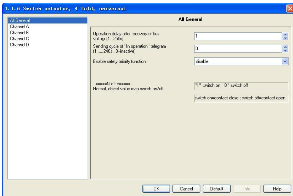
Fig.1 - Parameter window "All General"
